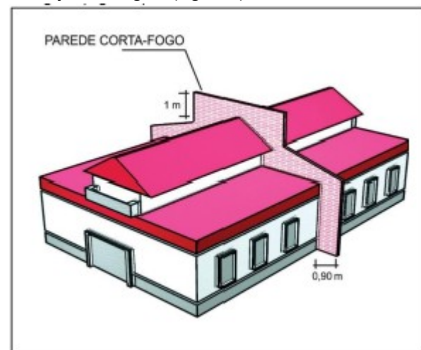
Figura 8: Parede corta-fogo
