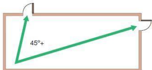
Figura nº 08: distância entre aberturas de saídas de emergência
